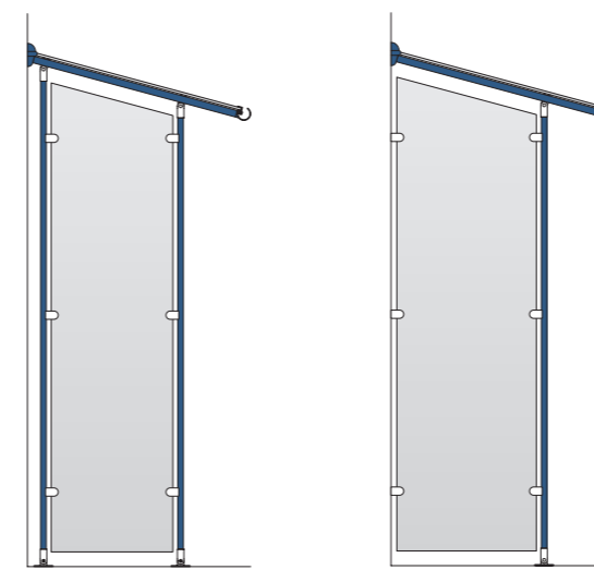
Typ WS
